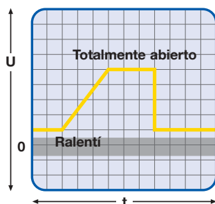
Potenciómetro de la válvula de mariposa imagen óptima
