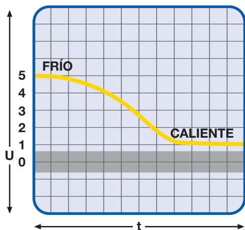
Figura 4: Sensor de temperatura del refrigerante
