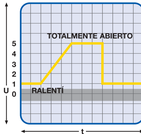
Figura 5: Potenciómetro de la válvula de mariposa
