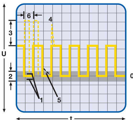
Figura 2: Oscilograma digital
