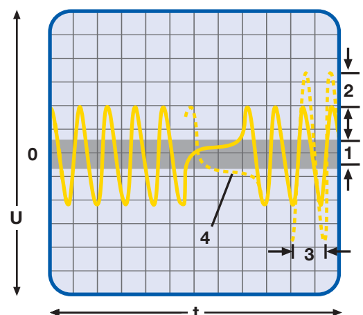
Figura 3: Oscilograma analógico
