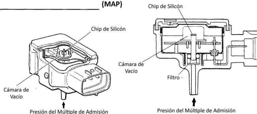
Sensor de Presión Absoluta del Múltiple (MAP)
