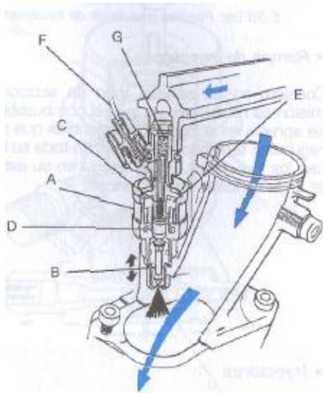
Figura 5.39. Inyector de un sistema de una Yamaha GTS 1000 c.c.
